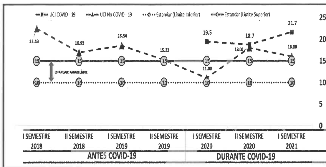
GRÁFICO N°9 : Promedio de Permanencia por Semestre del Pacientes COVID-19 o No COVID-19 ingresado a la UCI en el HNHU, periodo: 2018 – 2021
