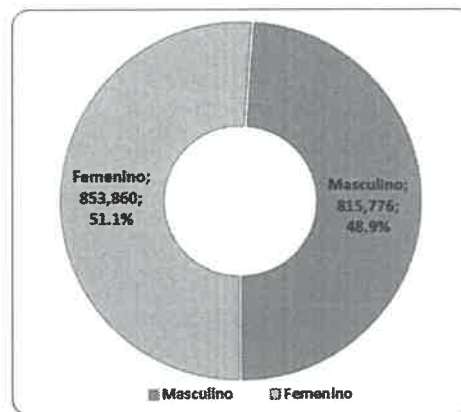
GRÁFICO N°2 : POBLACION PADRON TABLA N° 01 DIRIS LIMA ESTE – NOMINAL – INEI 2021 SEGÚN SEXO
