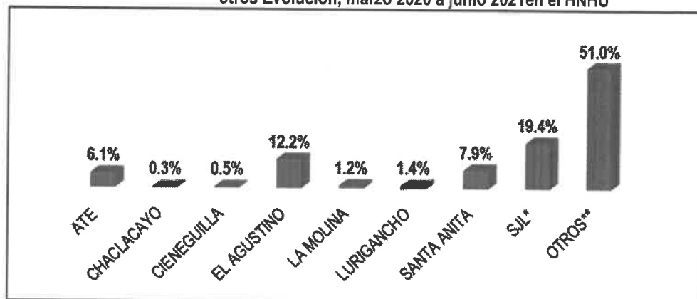
GRÁFICO N°11 : Procedencia de pacientes hospitalizados por la Covid-19 según distrito de la DIRIS LE y otros Evolución, marzo 2020 a junio 2021 en el HNHU
