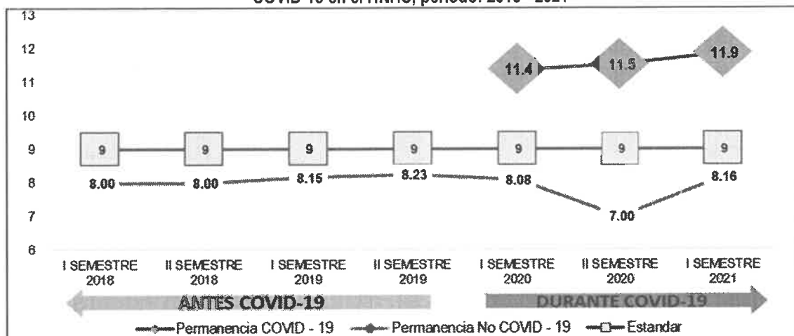
GRÁFICO N°12 : Promedio de Permanencia por Semestre Según Tipo de Pacientes COVID-19 o No COVID-19 en el HNHU, periodo: 2018 - 2021
