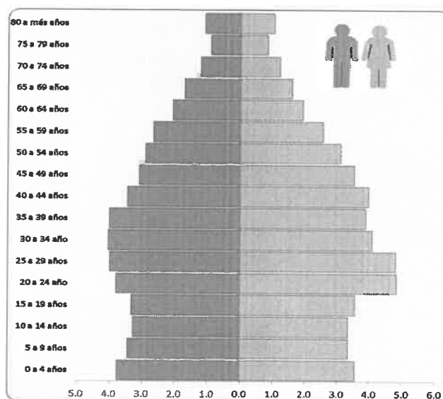
GRÁFICO N°3 : DIRIS LIMA ESTE: ESTRUCTURA GRUPO POBLACIONAL 2021 POR GRUPO ETAREO Y GENERO
