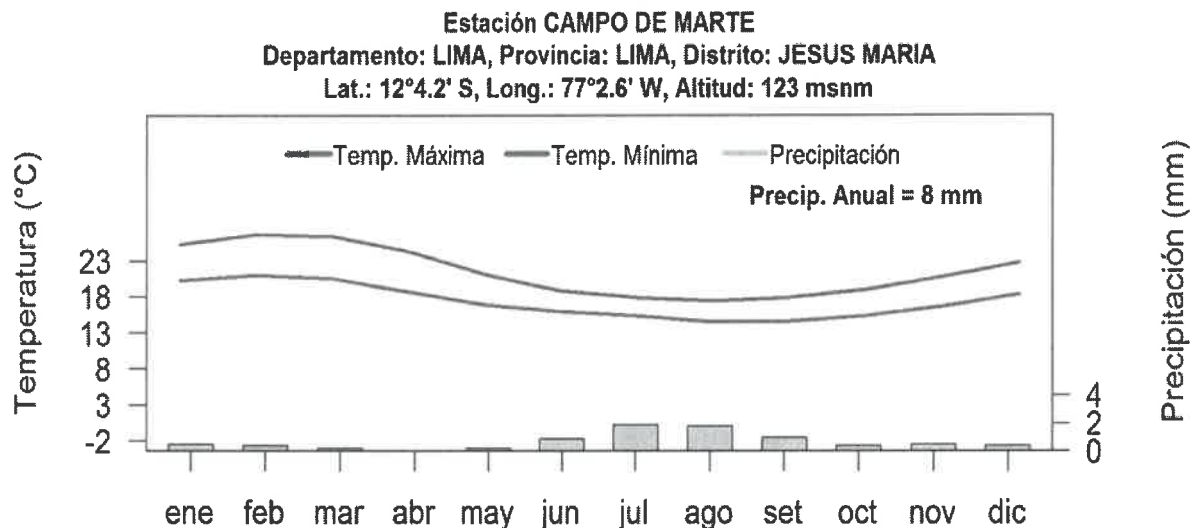
Gráfico N° 17 Distribución temporal de las temperaturas del aire y la precipitación en Campo de Marte
