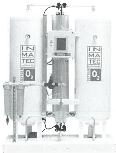
Imagen N°04 PGO marca INMATEC, Modelo POC 8400 med - HNHU, 2023
