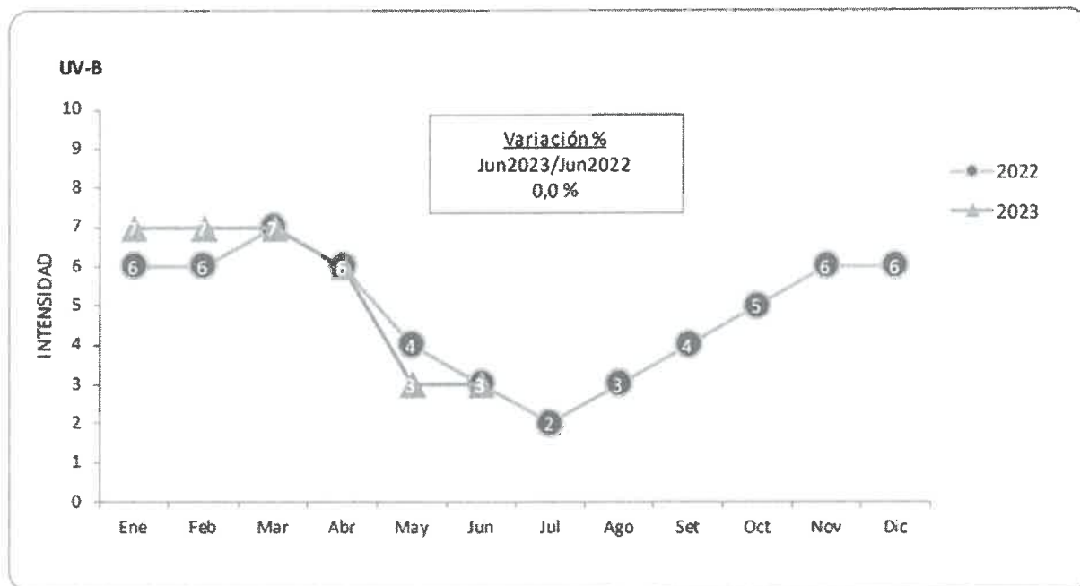
Grafico N° 18 Lima. Índice de radiación ultravioleta (IUV), según promedio mensual. Mes: junio 2022 / junio 2023
